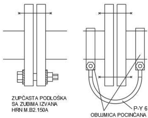
PRIRUBNICE (DETALJ)
